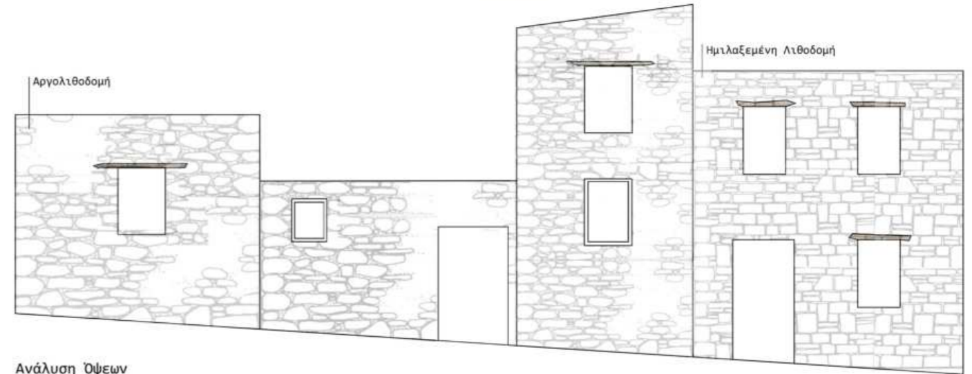
Ανάλυση Όψεων
